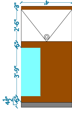
ELEVATION A
