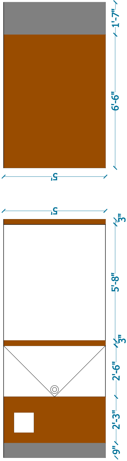
ELEVATION A
