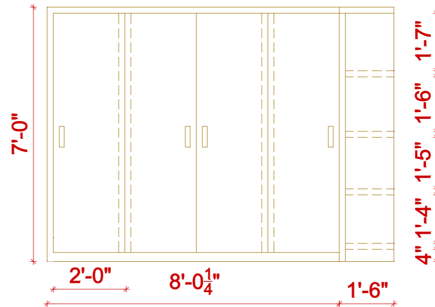
ELEVATION A
