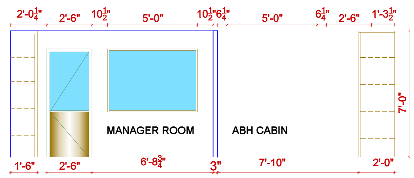
ELEVATION B
