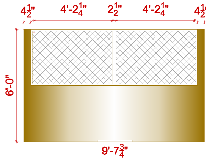
ELEVATION B
