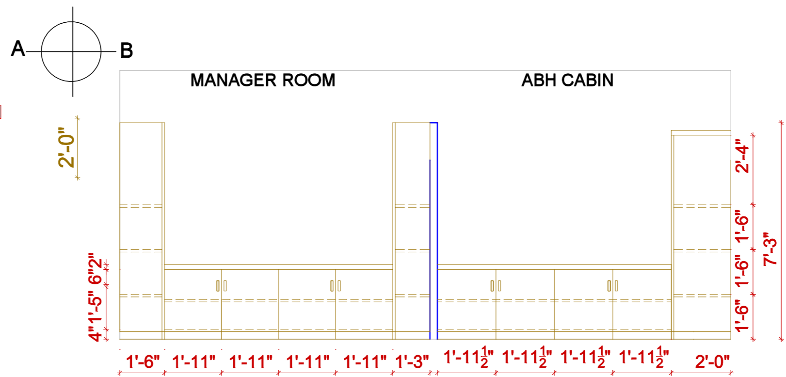
ELEVATION A
