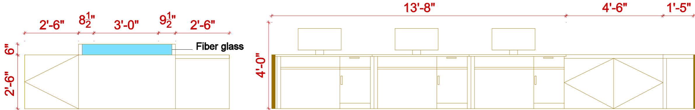
ELEVATION A
